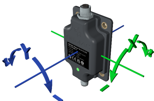
Abbildung 5: Ausrichtung x-up
