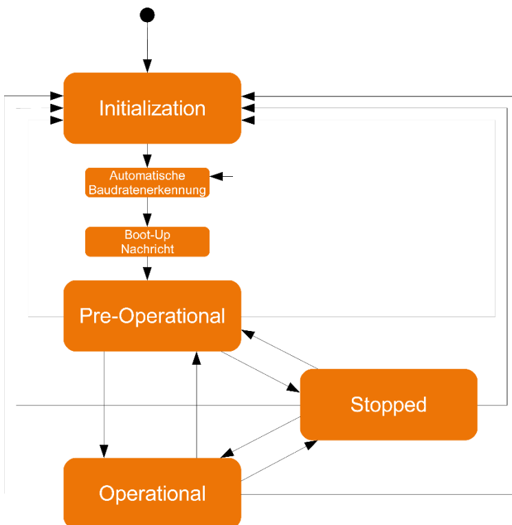
Abbildung 15: NMT Zustandsdiagramm
