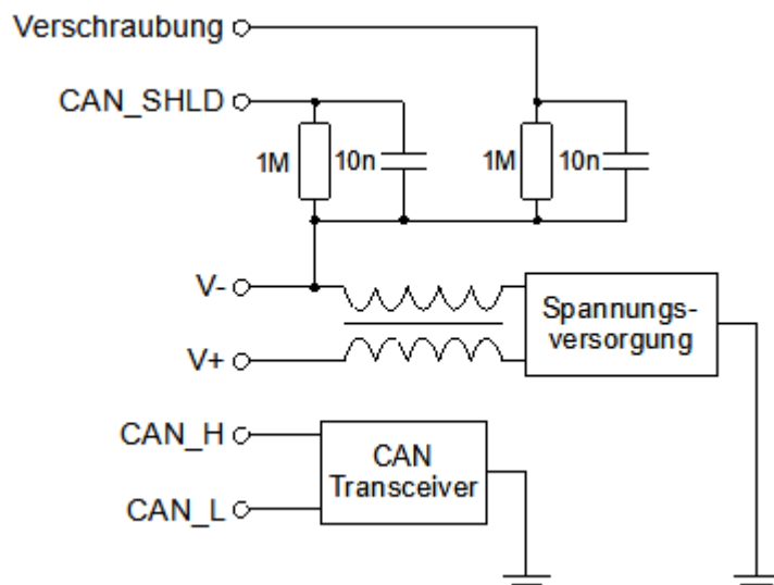
Abbildung 10: interne Beschaltung
