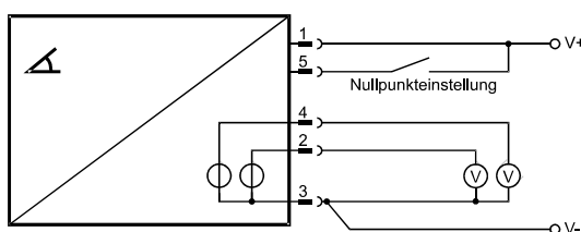
Spannungsschnittstelle
